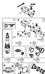
ETB-0000011490, Skrzynia biegów zewnętrzna hydrauliczna EA433 prawa
