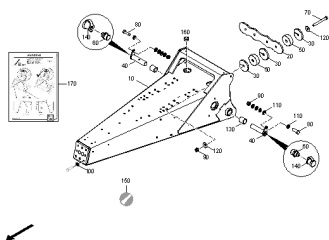
ETB-003416, Zawieszenie dolne dyszla
