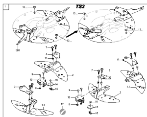
ETB-003442, Zestaw łopatek rozsiewających TS2
