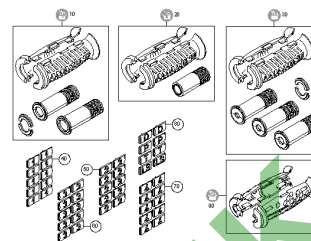
ETB-003466, Uchwyt węży hydraulicznego
