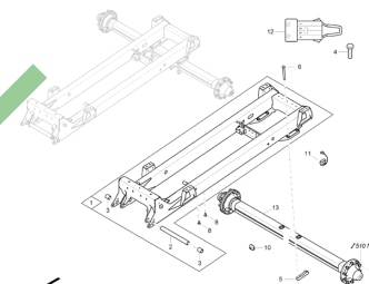
ETB-003426, Podwozie sztywne 2950 mm
