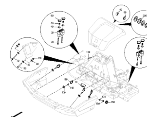
ETB-0000012285, Elementy złączne Auto TS i Flowcontrol z rynną skrętną TS
