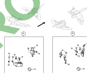
ETB-0000005223, Zestaw łopatek do rozsiewu granicznego TS30
