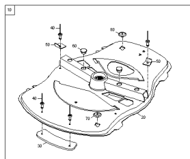
ETB-0000010282, Tarcza główna TS po lewej stronie przed
