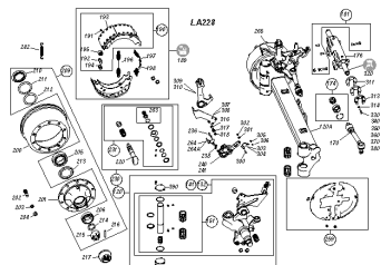
ETB-0000005354, Oś skrętna (LA228)
