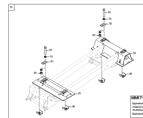
ETB-0000011914, Wsporniki montażowe
