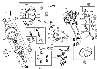
ETB-0000005354, Oś skrętna (LA228)
