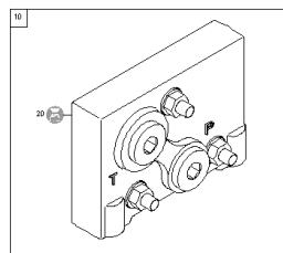
ETB-0000010678, Blacha końcowa
