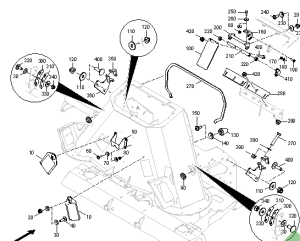
ETB-0000012004, System rozsiewania od 01.01.2025 (1)
