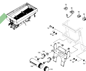
ETB-003412, 7501 / 10001 WAB, konstrukcja ciężarówki
