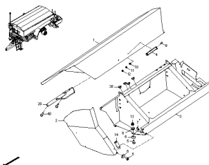
ETB-003420, Przednia skrzynia lewa (1)
