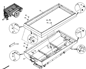
ETB-003410, Jednostka podstawowa 10001 do 31.12.2021
