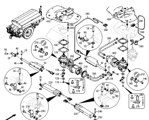
ETB-003438, Sterowanie przepływem napędu
