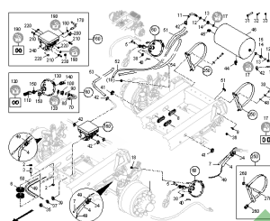
ETB-003430, Pneumatyczny układ hamulcowy (2)
