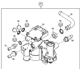
ETB-003433, Zawór hamulcowy przyczepy
