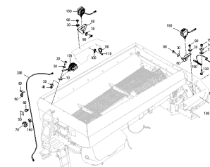
ETB-0000012040, Oświetlenie robocze od 01.01.2025
