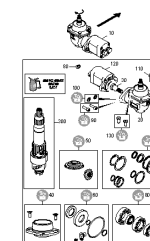
ETB-0000011492, Skrzynia biegów na zewnątrz hydraulicznie przełączana w prawo
