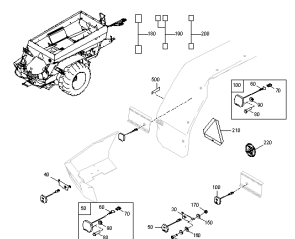
ETB-0000006089, Oświetlenie USA i Kanada
