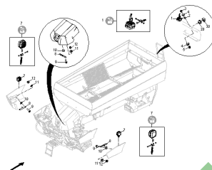
ETB-003463, Oświetlenie robocze
