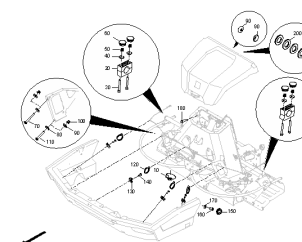
ETB-0000012285, Elementy złączne Auto TS i Flowcontrol z rynną skrętną TS
