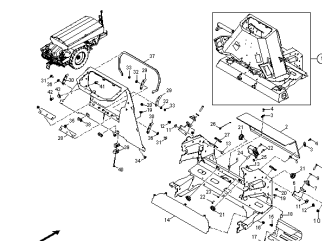
ETB-003473, Wspornik mechanizmu rozsiewającego (1)
