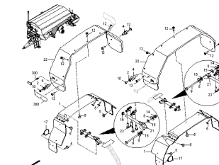
ETB-003436, Błotnik Vario
