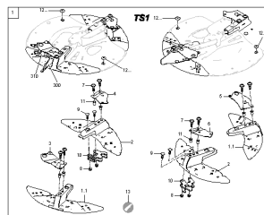
ETB-003439, Zestaw łopatek rozsiewających TS1
