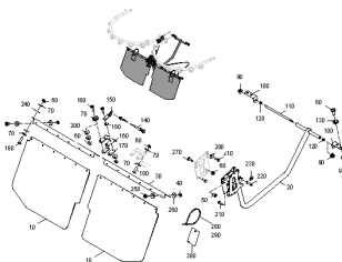
ETB-0000006054, Wspornik dyfuzora hydraulicznego (2)
