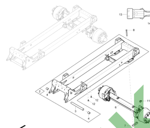
ETB-003425, Podwozie sztywne 2100 mm
