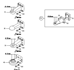
ETB-003417, Ucho pociągowe
