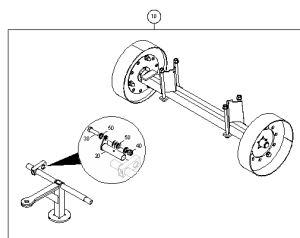
ETB-0000007472, Urządzenie manewrowe
