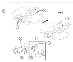
ETB-003440, Zestaw normalnych łopatek rozsiewających TS1
