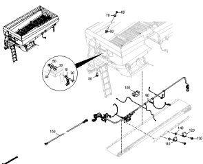
ETB-003459, Wiązka główna ZGTS-01
