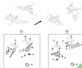
ETB-0000005219, Zestaw normalnych łopatek rozsiewających TS20
