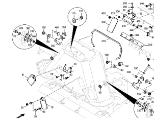
ETB-0000012004, System rozsiewania od 01.01.2025 (1)
