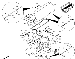
ETB-0000012270, Skrzynia transportowa po prawej stronie
