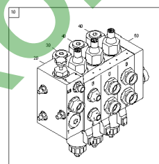
ETB-0000009988, Blok sterujący GD1034
