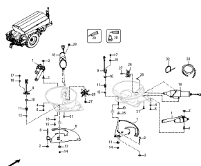
ETB-003468, Dno z otworami TS (2)
