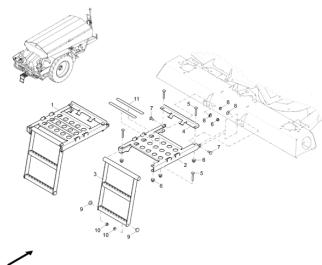
ETB-003471, Drabina mechanizmu rozsiewającego
