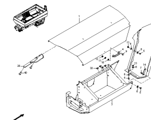
ETB-003423, Przednia skrzynia prawa (2)
