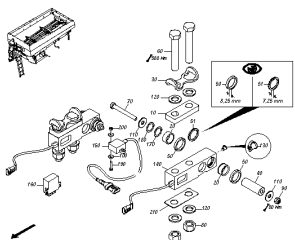
ETB-003428, System ważenia
