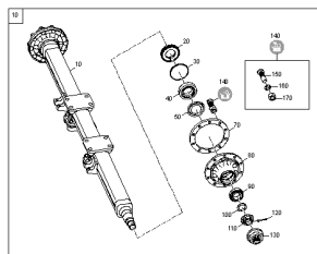
ETB-0000010334, Oś LA246
