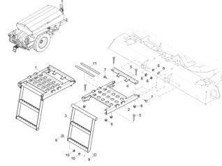
ETB-003471, Drabina mechanizmu rozsiewającego
