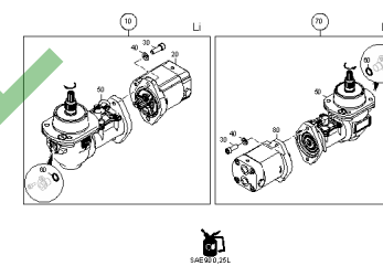
ETB-003452, Skrzynia biegów Hydro CFC
