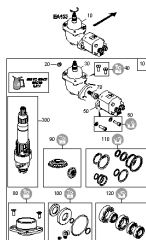
ETB-0000007183, Skrzynia biegów zewnętrzna hydrauliczna EA433 lewa
