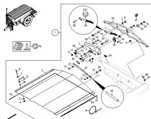
ETB-003483, Plandeka zwijana hydrauliczna (1)
