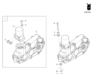
ETB-003481, Napęd taśmy
