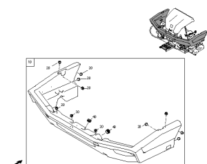
ETB-0000012000, Owiewka tylna od 01.01.2025
