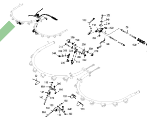
ETB-0000005411, Wspornik dyfuzora hydraulicznego (1)
