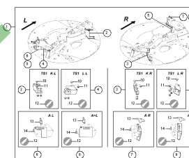
ETB-003441, Zestaw łopatek do rozsiewu granicznego TS1
