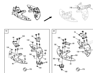
ETB-0000005215, Zestaw łopatek rozsiewających TS10
