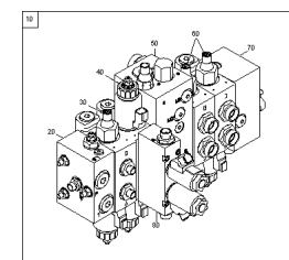
ETB-0000009991, Blok sterujący GD878
