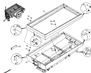
ETB-0000005506, Jednostka podstawowa 10001 od 01.01.2022
