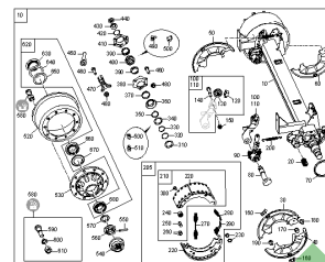
ETB-0000010335, Oś LA240 (1)
