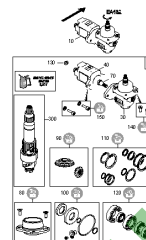
ETB-0000011490, Skrzynia biegów zewnętrzna hydrauliczna EA432 prawa
