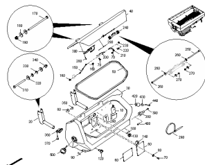
ETB-0000012278, Skrzynia transportowa lewa
