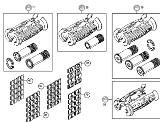
ETB-003466, Uchwyt węży hydraulicznego
