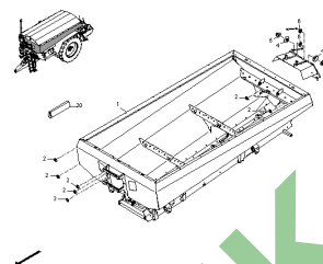
ETB-003411, Maszyna podstawowa 7501
