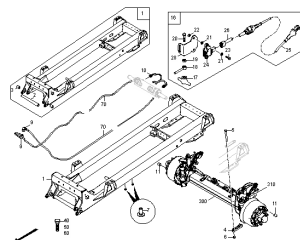
ETB-003424, Podwozie skrętnie 2100 mm
