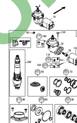
ETB-0000011491, Skrzynia biegów na zewnątrz hydraulicznie przesuwana w lewo
