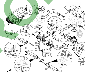
ETB-003438, Sterowanie przepływem napędu
