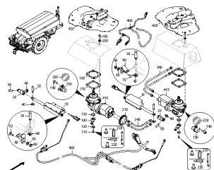
ETB-0000010278, Napęd samochodowy TS
