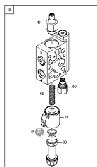
ETB-0000010677, Kierunkowy zawór sterujący Śmigłowiec Elektromagnes
