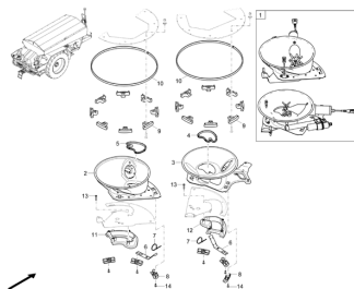
ETB-003467, Dno z otworami TS (1)
