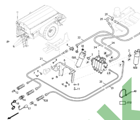
ETB-003451, Napęd hydrauliczny z układem kierowniczym
