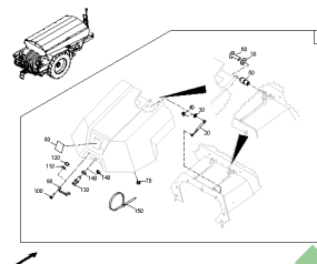
ETB-003472, Pokrywa mechanizmu rozsiewającego
