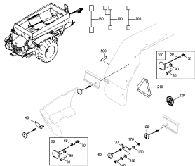
ETB-0000006089, Oświetlenie USA i Kanada
