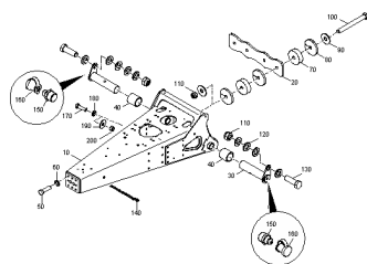
ETB-0000006768, Zaczep górny 2,5T
