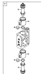
ETB-0000010680, Wegeventil Prop. Magnes
