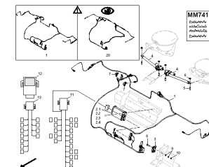
ETB-003465, Komponenty elektroniczne mechanizmu rozsiewającego
