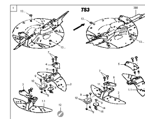
ETB-003445, Zestaw łopatek rozsiewających TS3
