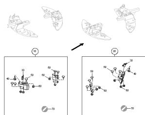
ETB-0000005217, Zestaw łopatek do rozsiewu granicznego TS10
