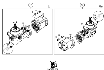
ETB-003452, Skrzynia biegów Hydro CFC
