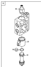
ETB-0000010675, Kierunkowy zawór sterujący Śmigłowiec Elektromagnes
