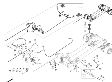
ETB-003435, Hydrauliczny układ hamulcowy (2)
