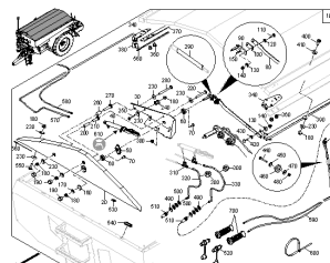
ETB-003485, Plandeka zwijana hydrauliczna (2)
