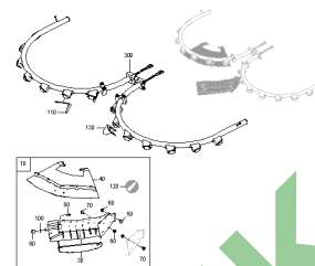
ETB-0000005413, Sito do rozrzucania na granicy
