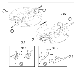
ETB-003443, Zestaw normalnych łopatek rozsiewających TS2
