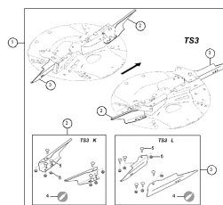
ETB-003446, Zestaw normalnych łopatek rozsiewających TS3
