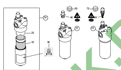
ETB-006791, Filtr hydrauliczny ciśnieniowy
