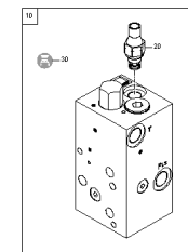
ETB-0000010681, Płyta pośrednia
