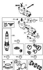
ETB-0000007183, Skrzynia biegów zewnętrzna hydrauliczna EA433 lewa
