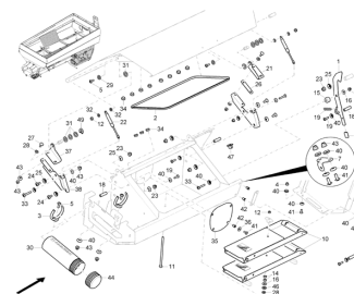
ETB-003422, Przednia skrzynia prawa (1)
