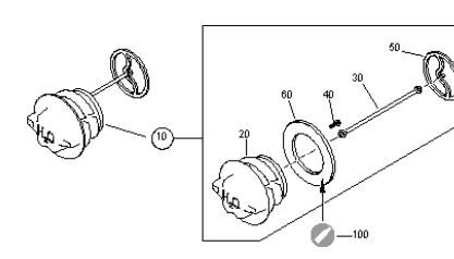
ETB-0000005951, Pokrywka z okrągłym gwintem
