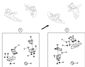
ETB-0000005216, Zestaw normalnych łopatek rozsiewających TS10
