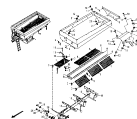
ETB-003482, Ruszty sitowe
