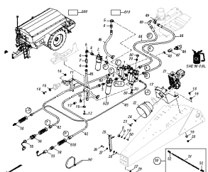
ETB-003455, Napęd Hybrid z układem kierowniczym
