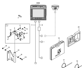
ETB-003479, Pakiet terminala Isobus CCI
