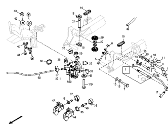
ETB-003432, Pneumatyczny układ hamulcowy (2)
