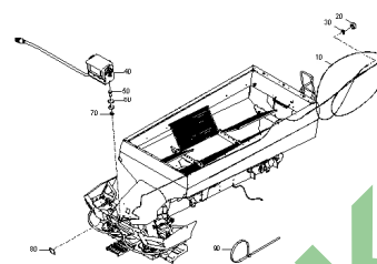
ETB-0000002686, Zestaw montażowy kamery cofania
