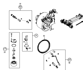
ETB-0000005355, Czujniki do LA228
