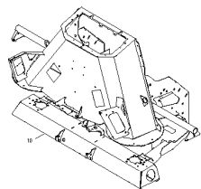
ETB-0000012031, Nośniki rozrzutników od 01.01.2025
