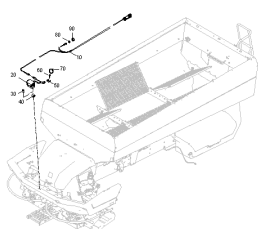
ETB-0000012042, Zestaw montażowy kamery cofania od 01.01.2025
