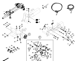
ETB-003429, Pneumatyczny układ hamulcowy (1)
