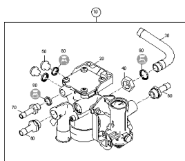
ETB-003433, Zawór hamulcowy przyczepy
