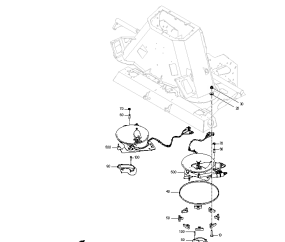
ETB-0000012019, System rozsiewania od 01.01.2025 (4)
