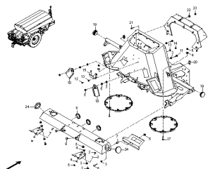
ETB-003474, Wspornik mechanizmu rozsiewającego (2)
