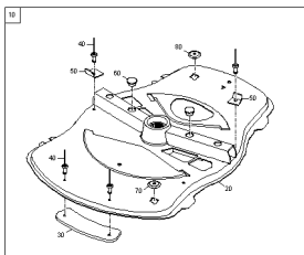
ETB-0000010282, Tarcza główna TS po lewej stronie przed
