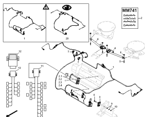
ETB-003465, Komponenty elektroniczne mechanizmu rozsiewającego
