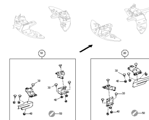
ETB-0000005216, Zestaw normalnych łopatek rozsiewających TS10
